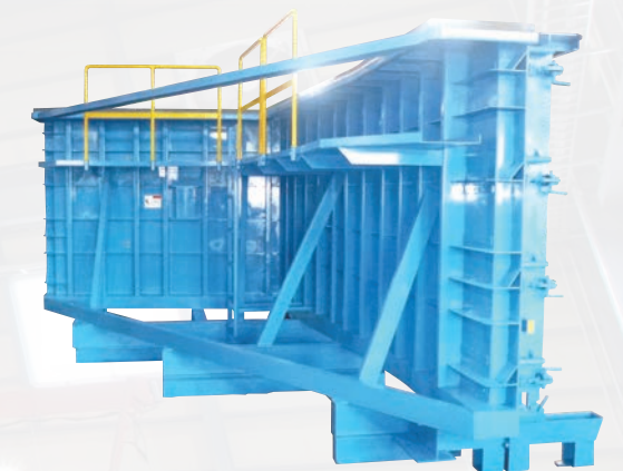
● L型擁壁(小口打)
